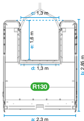
Recolector de alto rendimiento con paraguas delantero
