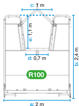
Recolector de aceituna con paraguas delantero Serie 100
