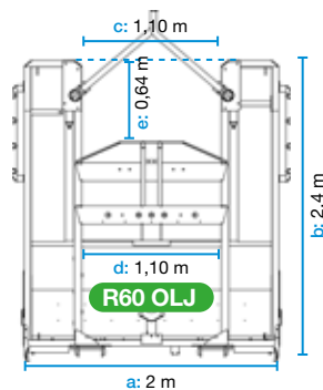
Recolector de alto rendimiento para olivo joven con paraguas delantero Serie 130. Vibración por circuito cerrado de pistones
